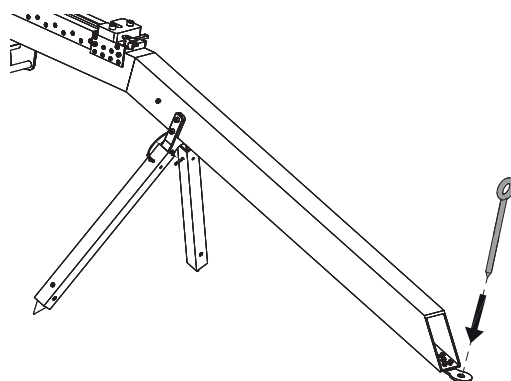
Фиксация хвостовика с помощью кола
