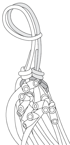
Петля кольца из синтетического троса
