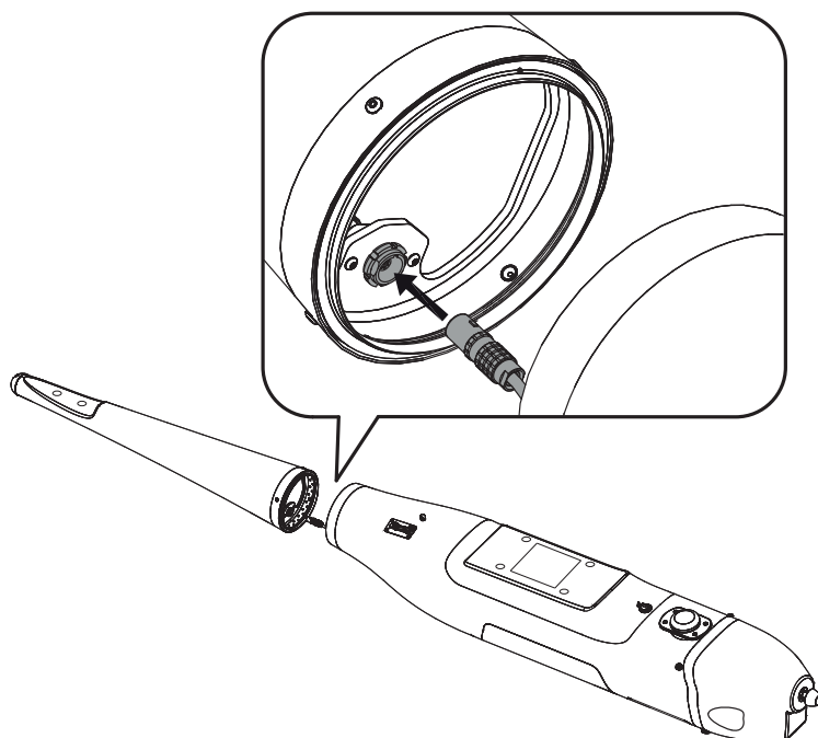
Подключение разъема хвостовой балки
