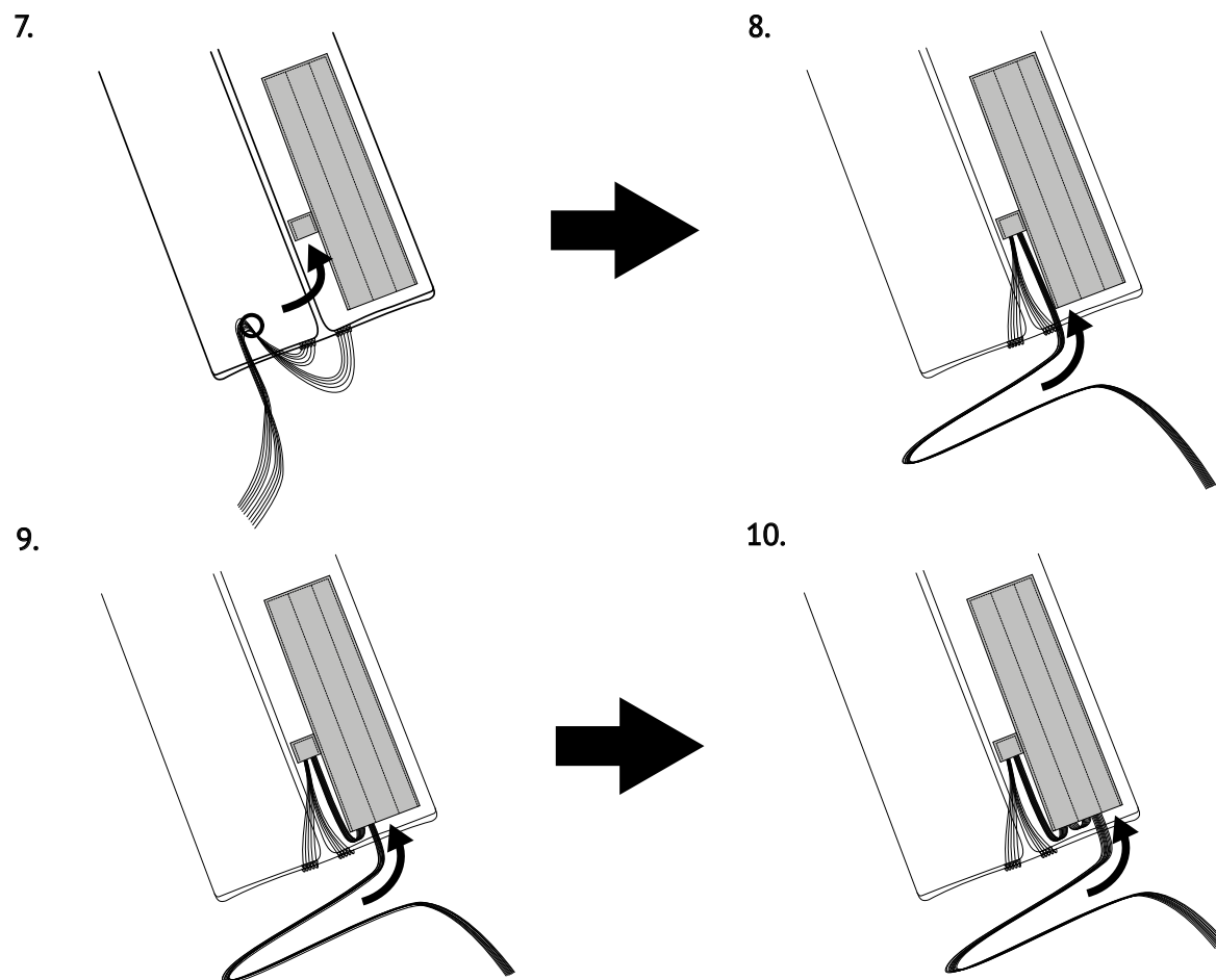
Укладка стопорного кольца и строп парашюта (шаги 7-10)
