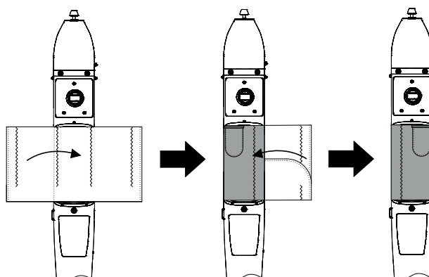
Укладка баллонета, ч.2
